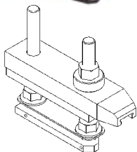
Bride de serrage rapide avec rainure T dans bloc réf. LP 001-335
